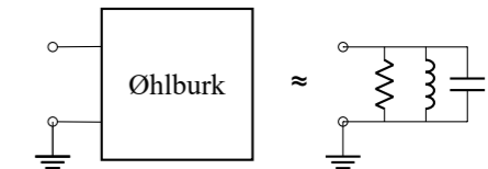
Figur 5. Enkel ekvivalent krets för en Øhlburk.
