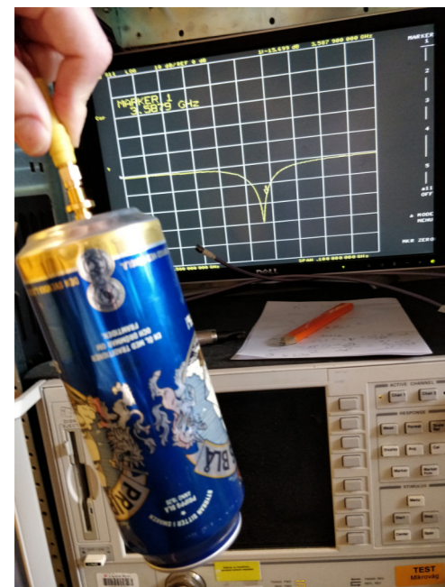
Figur 8. Långburk med matning på kortsidan
