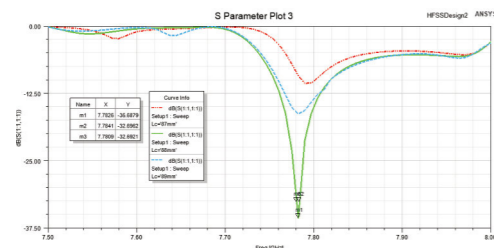
Figur 7. S_{11} av den simulerade kortburken samt närliggande längder på matrelementet.
