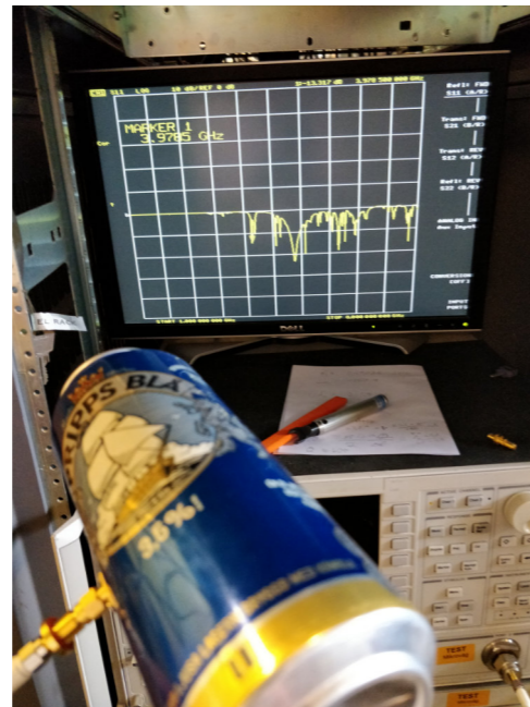
Figur 9. Långburk med matning på långsidan
