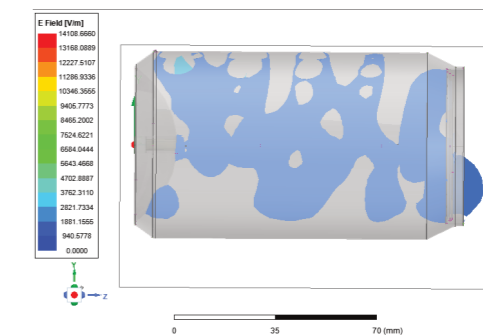
Figur 6. Simuleringsmodell med E-fältet utritat vid en fasvinkel på 90deg. Notera hur elektronerna rymmer från öppningen av burken. Ineffekt 0dbm
