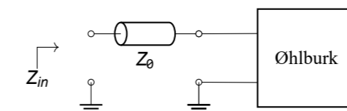
Figur 4. Tvåportdefinition.
